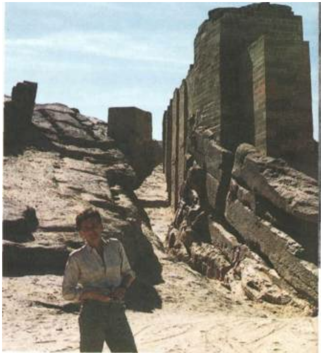
No açude sul da barragem, as fundações de um muro monolítico foram fixadas no rochedo.
